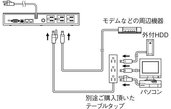
電源出力コンセント
