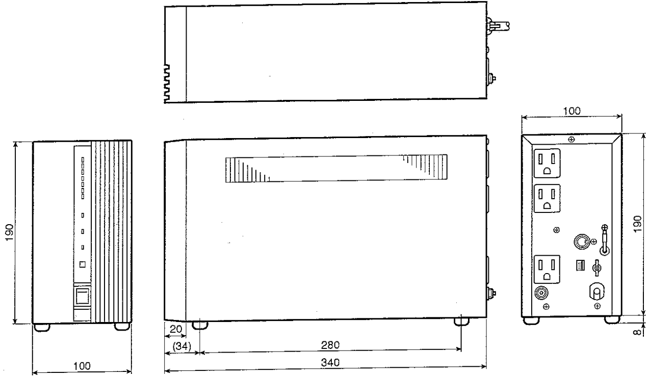
BU504XIV寸法図
