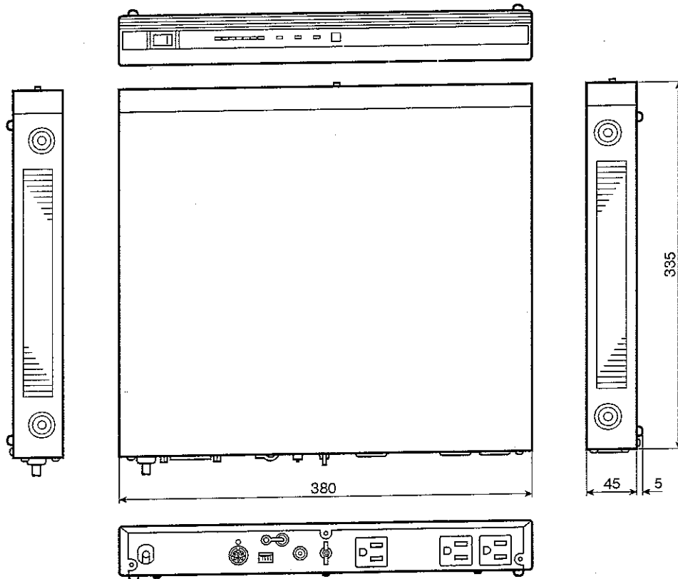
BU504XLIV寸法図
