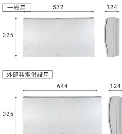
V2X用全負荷分電盤
